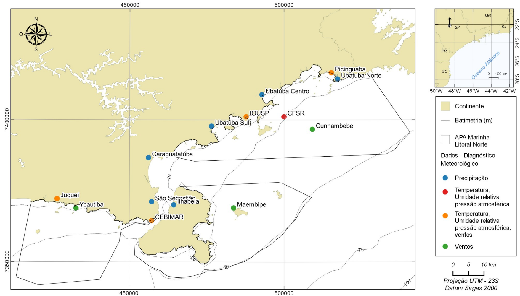
Figura 2.2.1.1-2 – Locais de obtenção dos dados utilizados na caracterização Climática e Meteorológica da APAMLN.
