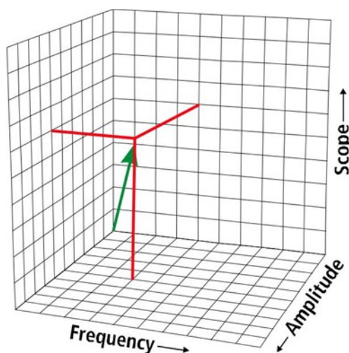
Figura 2.2.1.3.3-7 – Modelo conceitual do Índice de Qualidade de Águas Costeiras (IQAC).
