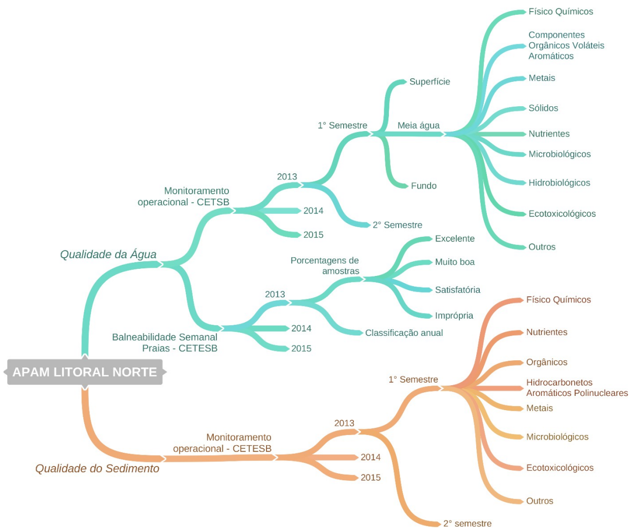
Figura 2.2.1.3.3-6 – Dados utilizados para o diagnóstico de qualidade de água e sedimento na APAMLN e entornos. Os grupos de compostos analisados estão apresentados somente para o ano 2013 no 1º semestre, porém, são representativos também para o 2º semestre de 2013 e para os anos de 2014 e 2015 (1º e 2º semestres) e em todas as profundidades (qualidade de água – monitoramento operacional CETESB).
