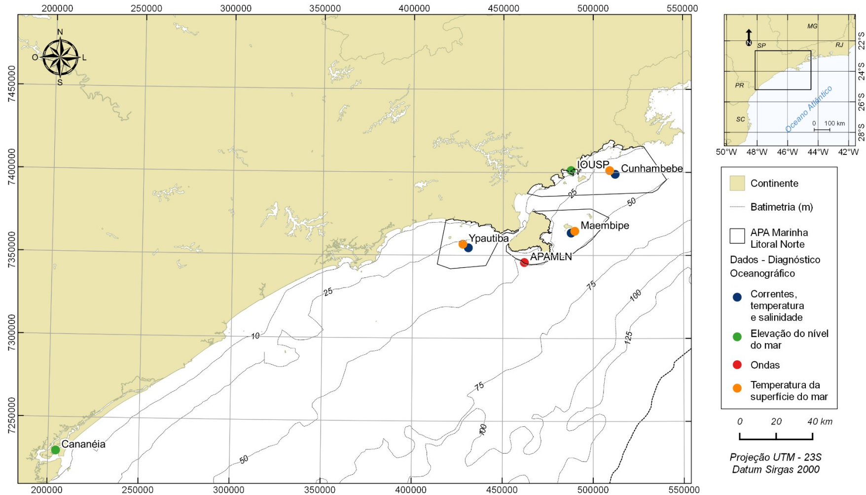
Figura 2.2.1.3.2-5 – Localização dos pontos de obtenção de dados utilizados no diagnóstico oceanográfico para a APAMLN
