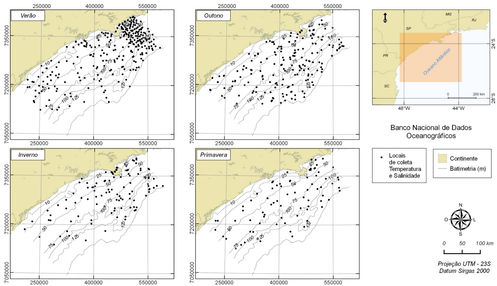
Figura 2.2.1.3.2-4 – Locais de coleta de dados de temperatura e salinidade obtidos junto ao Banco Nacional de Dados Oceanográficos. Os painéis superiores mostram dados coletados no verão (esquerda) e outono (direita) e os inferiores no inverno (esquerda) e primavera (direita).
